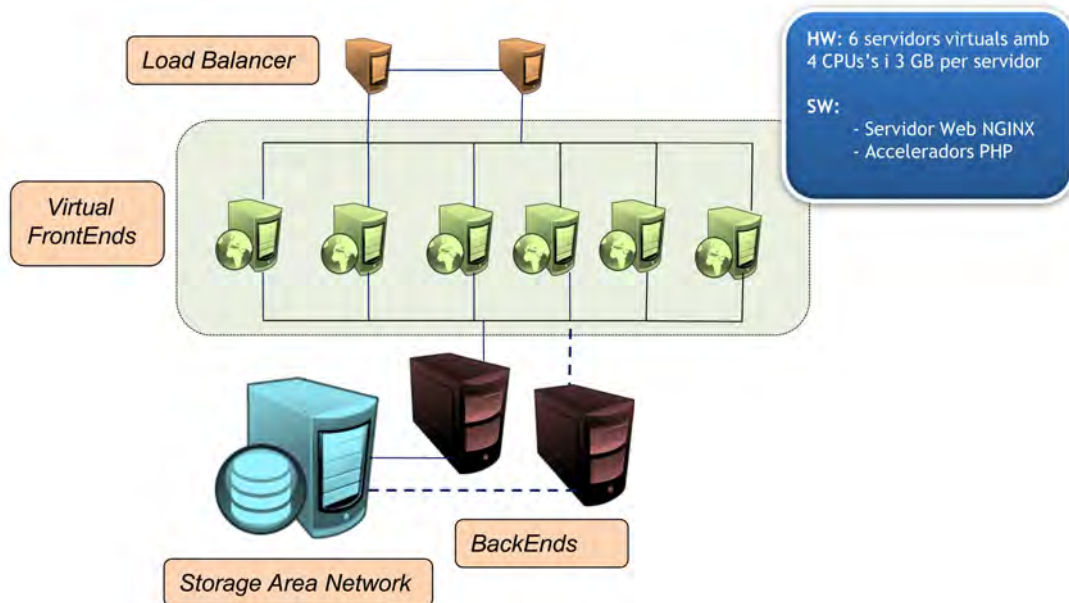
Arquitectura ATENEA
